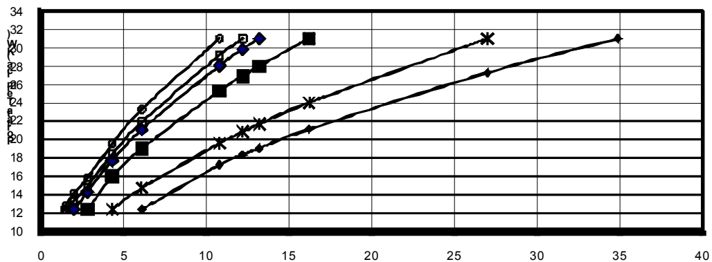
2.11.1 DIAGRAMMA PRESSIONE GAS - PORTATA TERMICA
