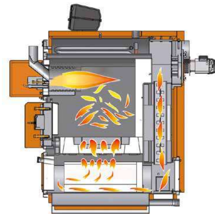
SEZIONE CALDAIA
